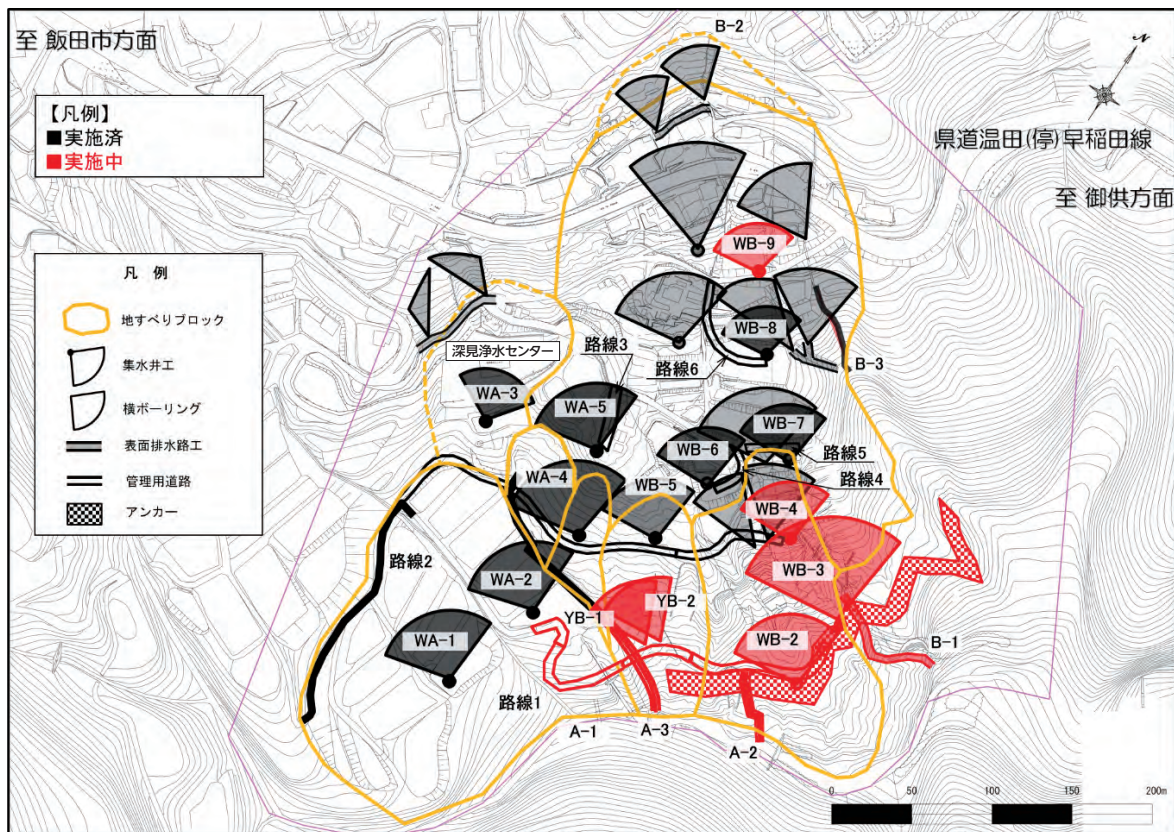
集水井工全体(イメージ)
